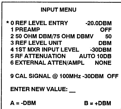
Figure 4-2. The Input Menu.
